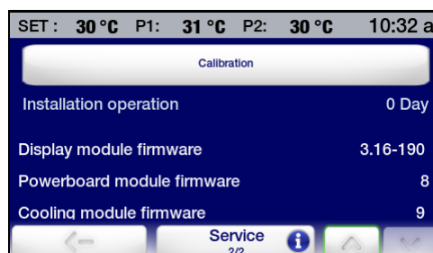
Página 2
