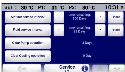
Página 1
