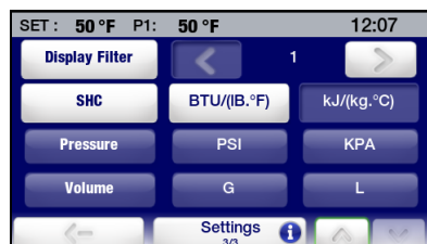
Preferencias – Página 3
